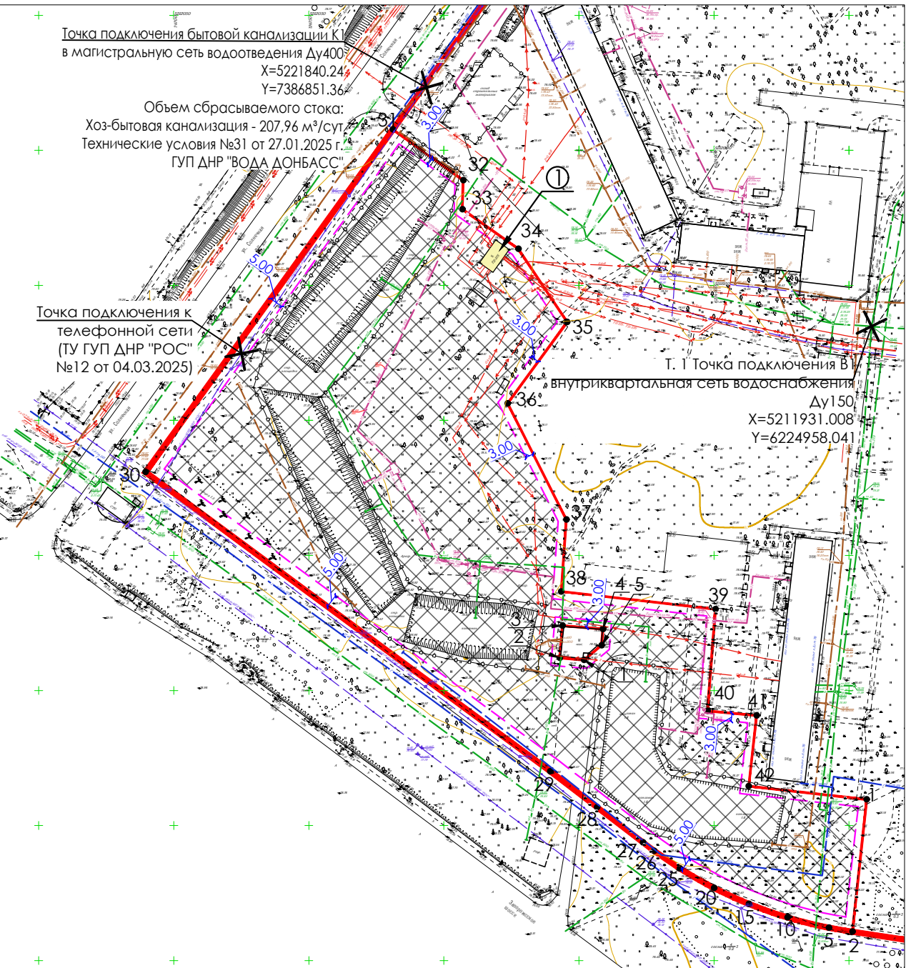
Чертеж градостроительного плана земельного участка разработан на топографической съемке, М1:2000
