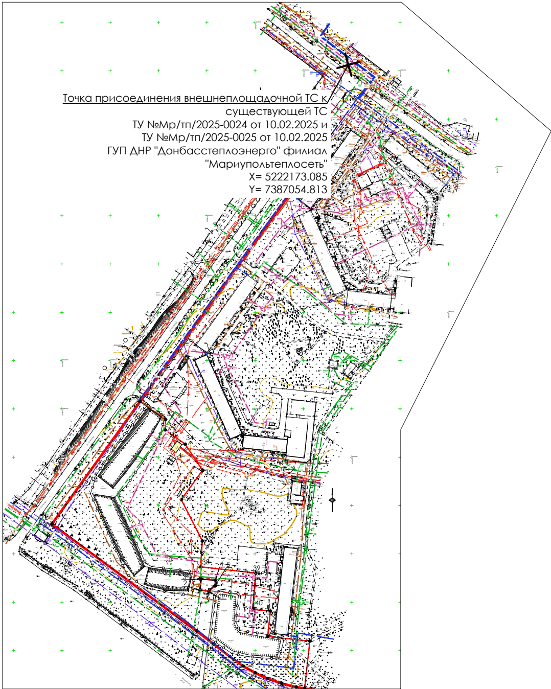
Чертеж точки подключения теплосети 1:4000
